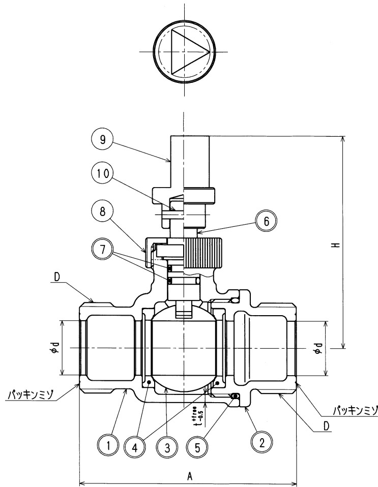
寸法表 (mm)
